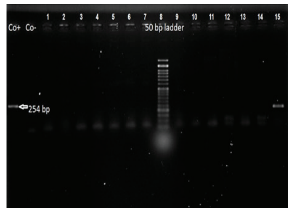
تصویر ۲- نتایج PCR برای شناسایی ژن aggR. از سمت چپ نخستین چاهک نمونه کنترل مثبت (سویه EAEC17-26)، دومین چاهک کنترل منفی و آخرین چاهک نمونه مثبت برای ژن aggR است.
