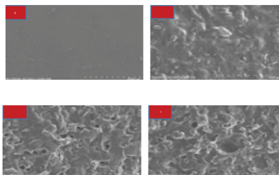
شکل ۱- تصویر MES در ابعاد ۵۰۰ میکرومتر از (الف) نمونه کنترل، (ب) نمونه ۱۰ درصد، (ج) نمونه ۲۰ درصد و (د) نمونه ۴۰ درصد
