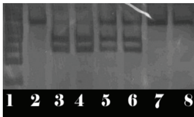
شکل ۱- نتیجه الکتروفورز محصول PCR در موقعیت A/T 251
