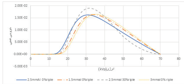
شکل ۴: طیف اشعه ایکس به دست آمده از برنامه SRS-78
