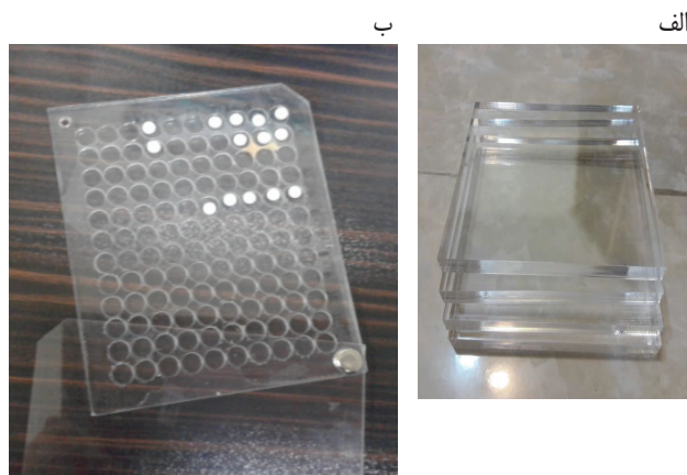
شکل ۳: الف) پلکسی به ابعاد ۱۰×۱۰×۱ سانتی متر، ب) چپیس ای TLD برای تعیین دوز در سطوح فانتوم
