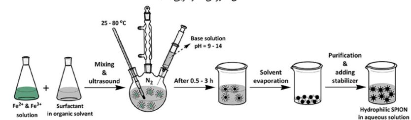
شکل ۵. روش میکروامولسیون (۶۸)
