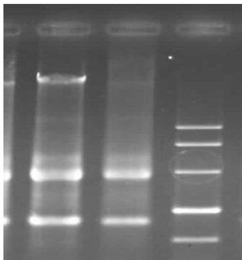
شکل ۱- الکتروفورز ژل آگارز برای نمونه‌های RNA استخراج شده است. وجود دو باند ۱۸S و ۲۸S روی ژل مشخص‌کننده کیفیت مطلوب RNA است.
