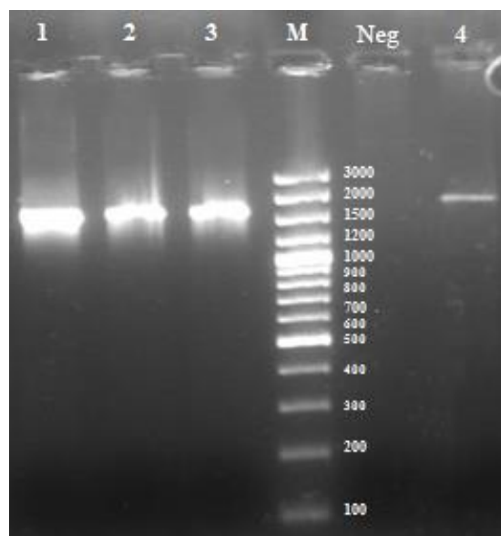
شکل ۲- الکتروفورز ژل آگارز محصول PCR ناحیه 16S rRNA: ۱، ۲) استافیلوکوکوس اپیدرمیدیس، ۳) استافیلوکوکوس هومینیس، ۴) باسیلوس سوبتیلیس، M) نشانگر اندازه ۱۰۰ جفت باز، Neg) کنترل منفی
