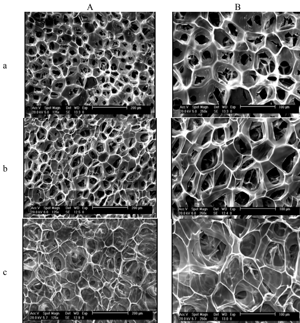
شکل ۱- میکروگراف های الکترونی داربست های کیتوزان-ژلاتین ایجاد شده در دمای ۲۰- و در زمانهای (a) ۲۰، (b) ۲ و (c) ۲۴ ساعت از مرحله پیش انجامد. بزرگنمایی تصاویر ستون (A) 125 X، (B) 250 X.
