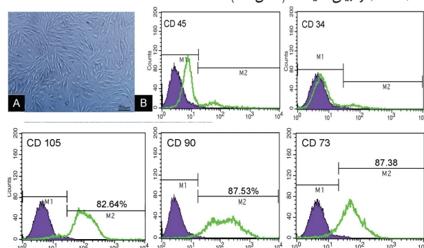
شکل ۱: ویژگی‌های سلول‌های بنیادی مزانشیمی مغز استخوان انسان در پاساژ چهارم. (A) تصویر میکروسکوپی سلول‌های مزانشیمی که ظاهر یکدست، دوکی شکل و شبه فیبروبلاست آن‌ها را نشان می‌دهد. (B) نمودارهای فلوسایتومتری نشان می‌دهد که این سلول‌ها شاخص‌های سطحی مزانشیمی شامل CD90، CD105، و CD73 را با درصد بالا بیان می‌کنند، درحالی‌که شاخص‌های سلول‌های خونساز CD34، CD45 را بیان نمی‌کنند.
