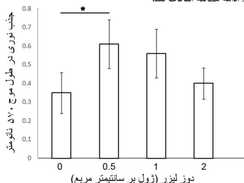
شکل ۲: نمودار حاصل از آزمایش MTT برای تعیین دوز مناسب لیزر کم‌توان هلیوم-نئون. همان‌طور که مشاهده می‌شود دوز لیزر ۰/۵ ژول بر سانتی‌متر مربع به‌طور معناداری موجب افزایش تکثیر فیبروبلاستها شده است. به طوری که میزان جذب نوری این گروه 0.13 \pm 0.06 بود، درحالی‌که جذب نوری گروه تیمار نشده با لیزر 0.11 \pm 0.03 است. نتایج مربوط به سه بار تکرار است، داده‌ها به صورت میانگین \pm انحراف معیار ارائه شده و علامت ستاره نشانه اختلاف معنادار در سطح p < 0.05 است.
