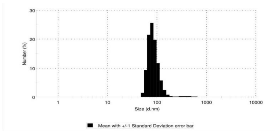
شکل ۳ نتایج به دست آمده از آنالیز DLS با استفاده از دستگاه MALVERN که محدوده اندازه اگزوزوم ها تعیین شده است.
