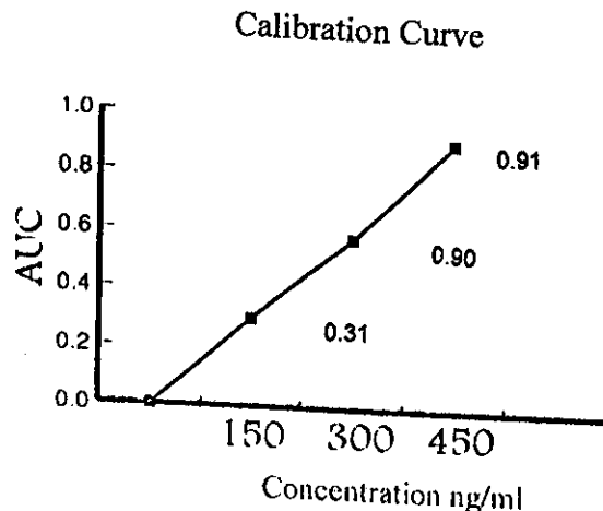
نمودار ۱: منحنی کالیبراسیون در روش LLE در غلظت‌های ۱۵۰، ۳۰۰ و ۴۵۰ نانوگرم بر میلی‌لیتر کدئین
