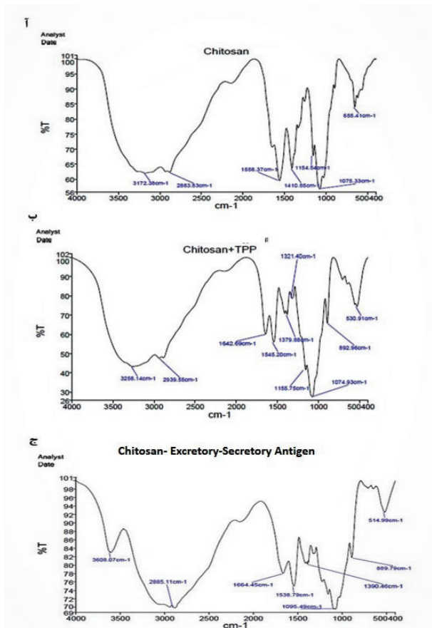
شکل ۳. آنالیز FTIR: (A) نانوذره کیتوزان، (ب) کیتوزان + TPP، (ج) کیتوزان همراه شده با آنتی ژن ترش‌جی-ترش‌جی
