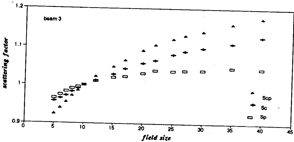
شکل ۴- Scp, Sc و Sp برای پرتوهای ^{60}\text{Co} و پرتو PMV (a, b) و (c)
